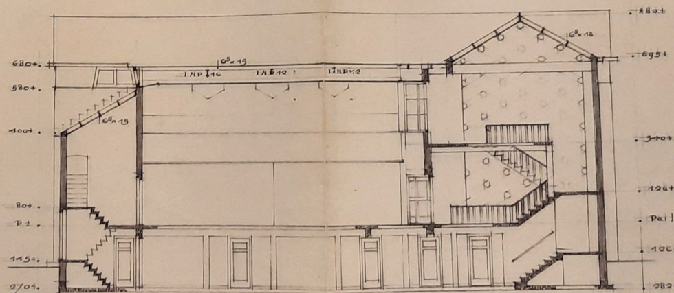
DOORSNEDE C-C
