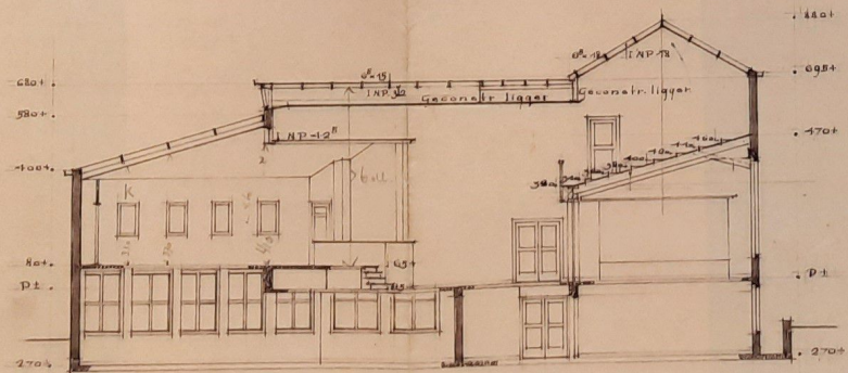
DOORSNED E A-A
