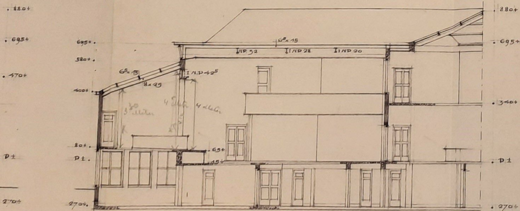
DOORSNEDE B-B
